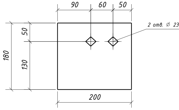
Дет. 1098
