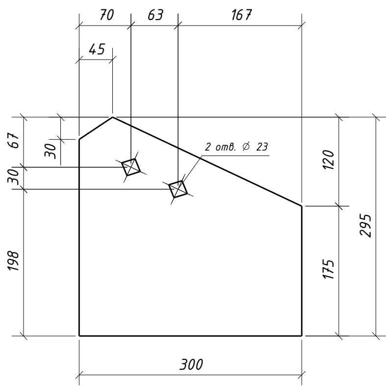
Дет. 123
