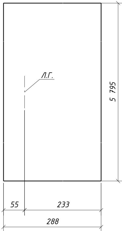
Развертка дет. 1249
