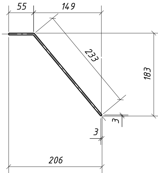
Гиб дет. 1249
