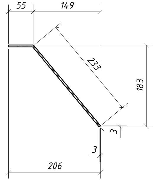
Развертка дет. 1251
