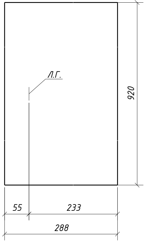
Развертка дет. 1251
