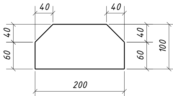
Дет. 202
