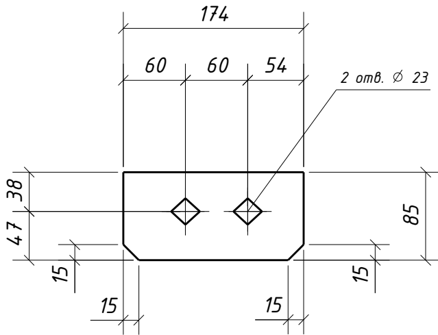
Дет. 226
