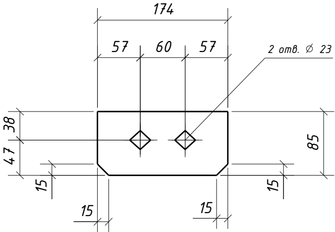
Дет. 227
