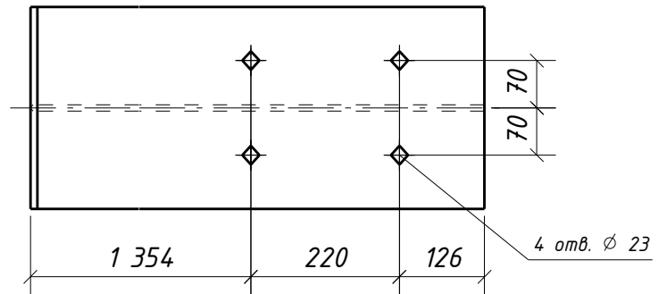
Вид снизу
