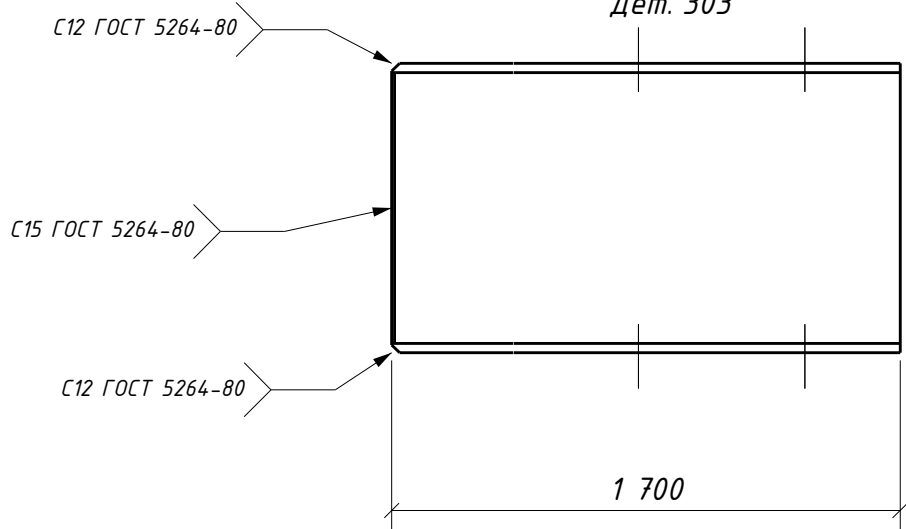
Дет. 303
