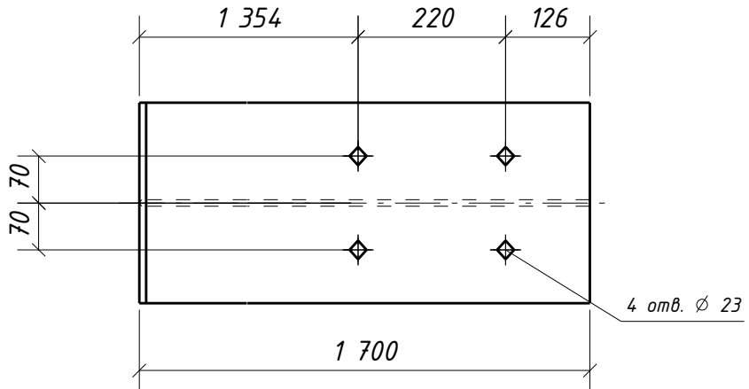
Вид сверху
