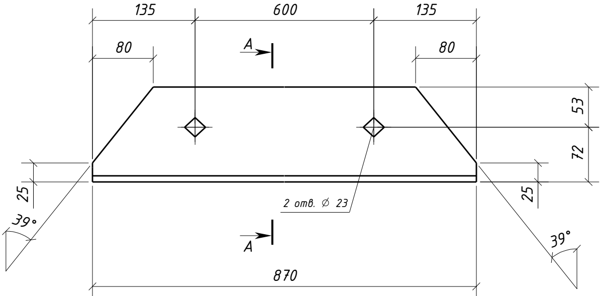
Дет. 521
