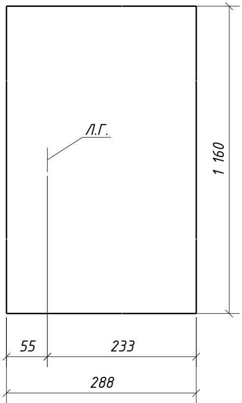
Развертка дет. 628
