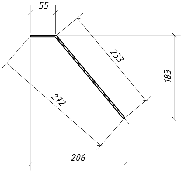
Гиб дет. 628
