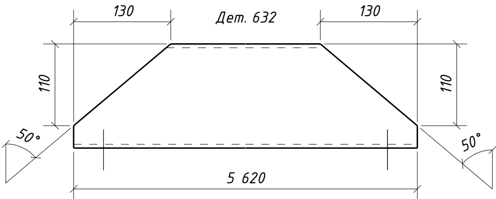
Дет. 632 2 отв. \varnothing 19
