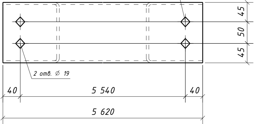
Дет. 632 2 отв. \varnothing 19
