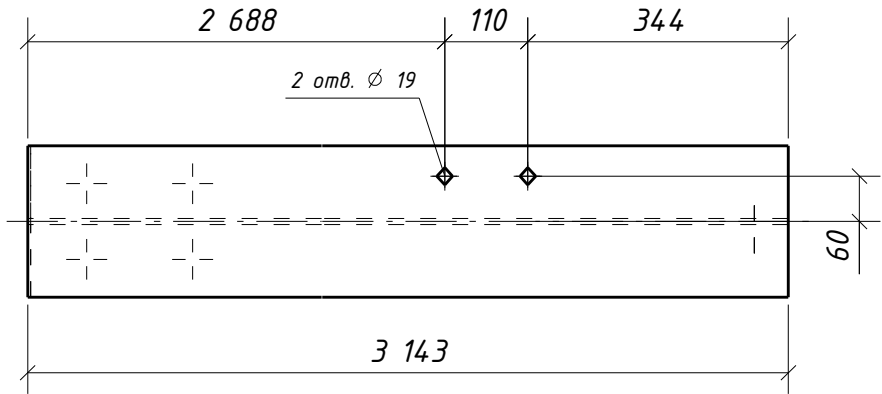
Вид сверху
