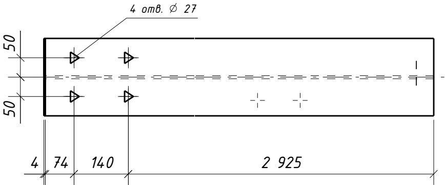
Вид снизу
