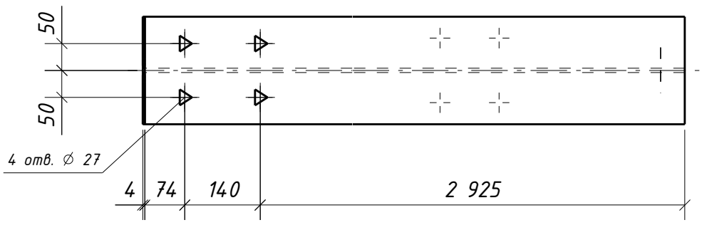
Вид снизу
