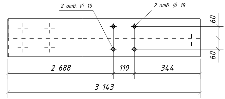
Дет. 91
