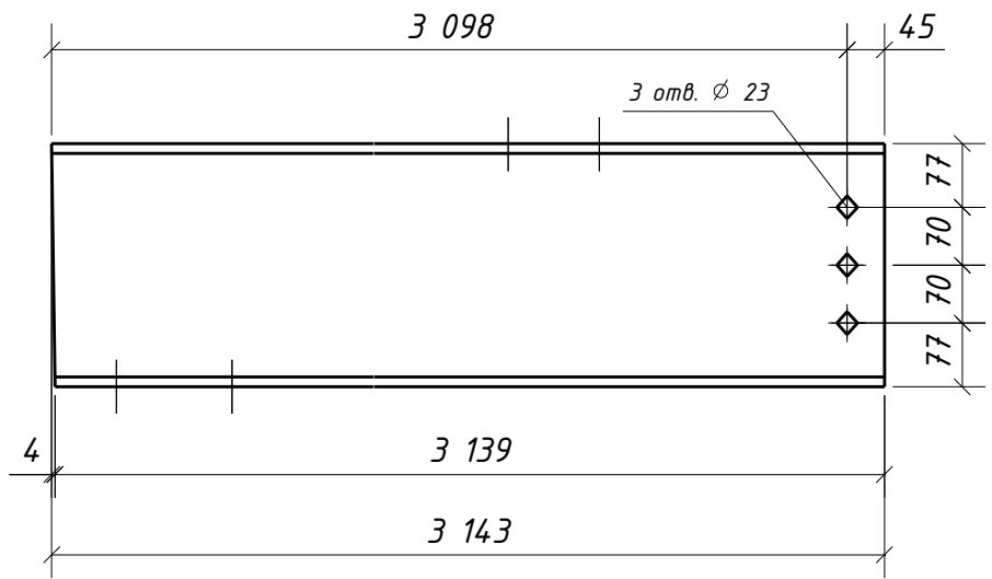
Дет. 91
