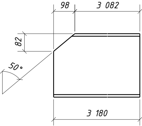
Дет. 92
