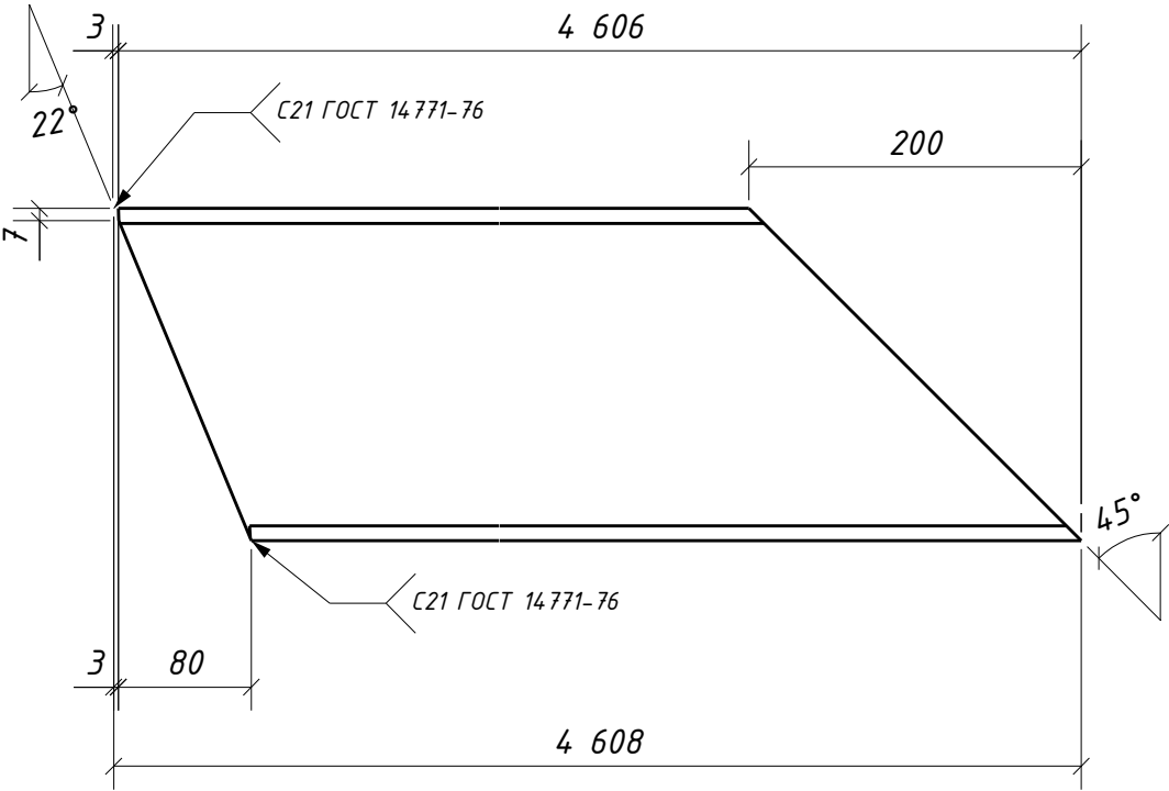
Дет. 1206
