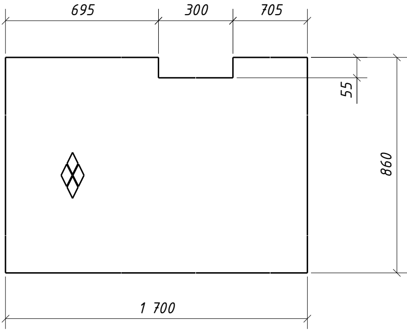
Дет. 1379
