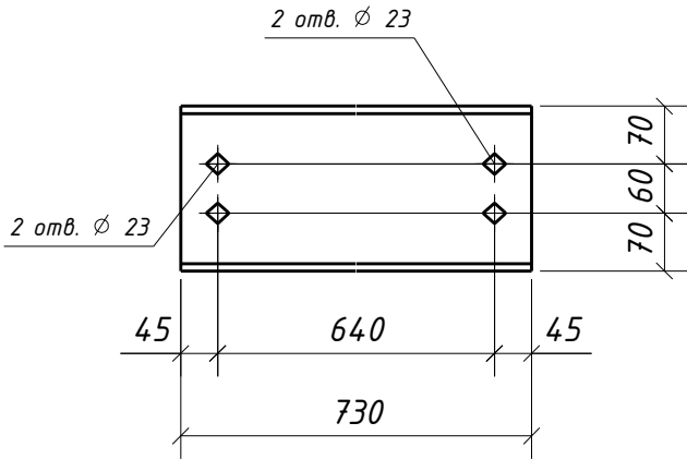
Дет. 1696
