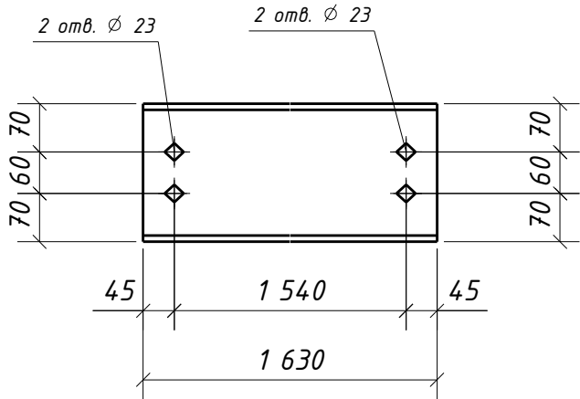
Дет. 1697
