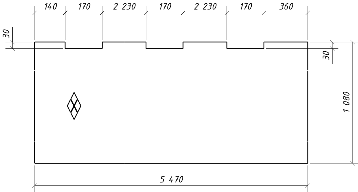
Дет. 1802
