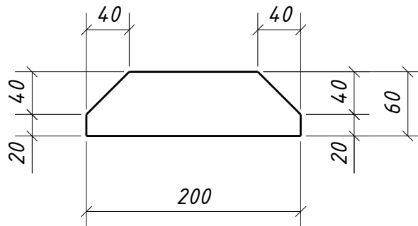
Дет. 203
