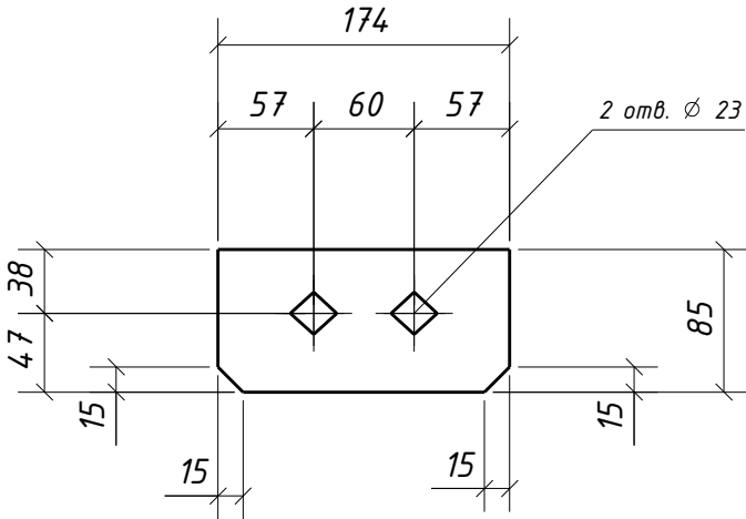
Дет. 227
