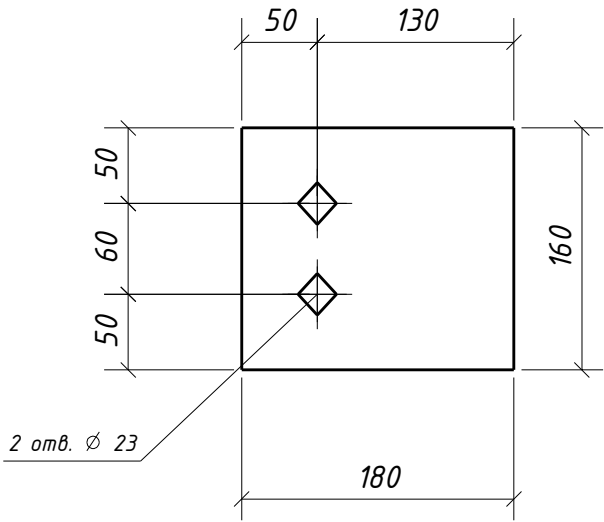
Дет. 232
