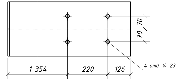
Вид снизу
