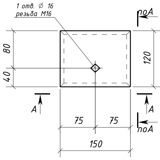
Дет. 504
