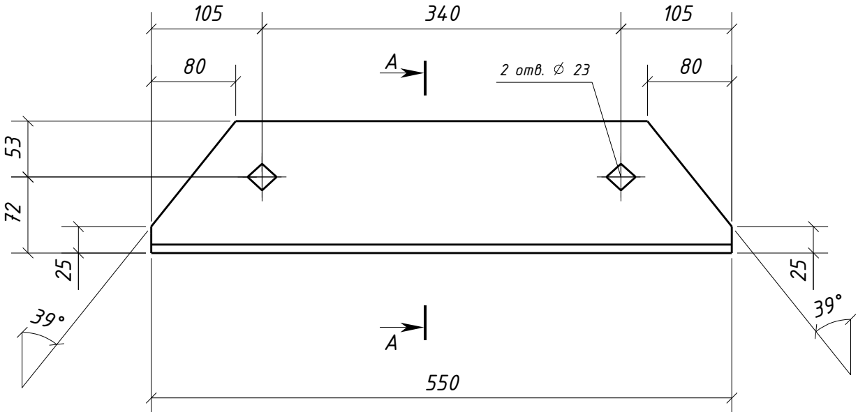
Дет. 522
