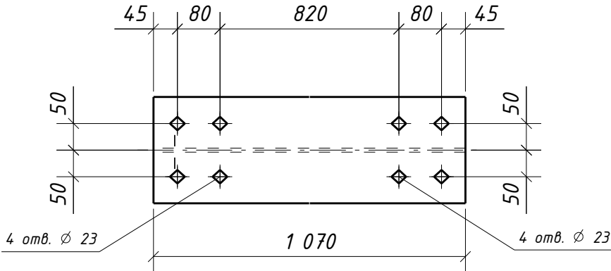
Дет. 93
