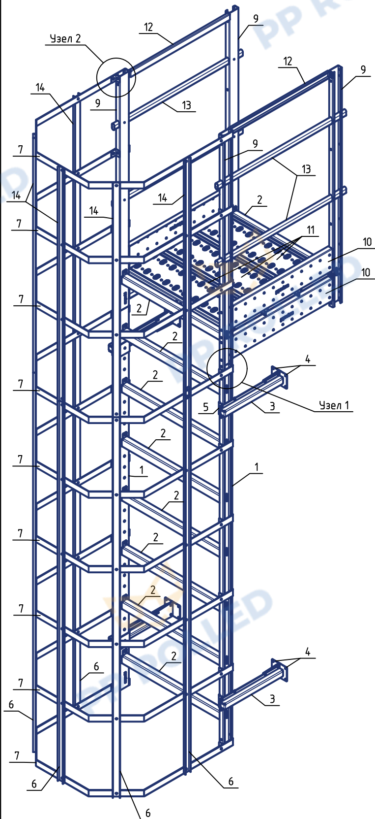
Сборная пожарная лестница П1-2 Н=2450 Общий вид
