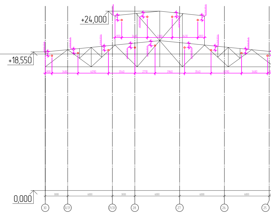
Рарзер 2-2. Расположение лучей С2000-ИПДЛ
