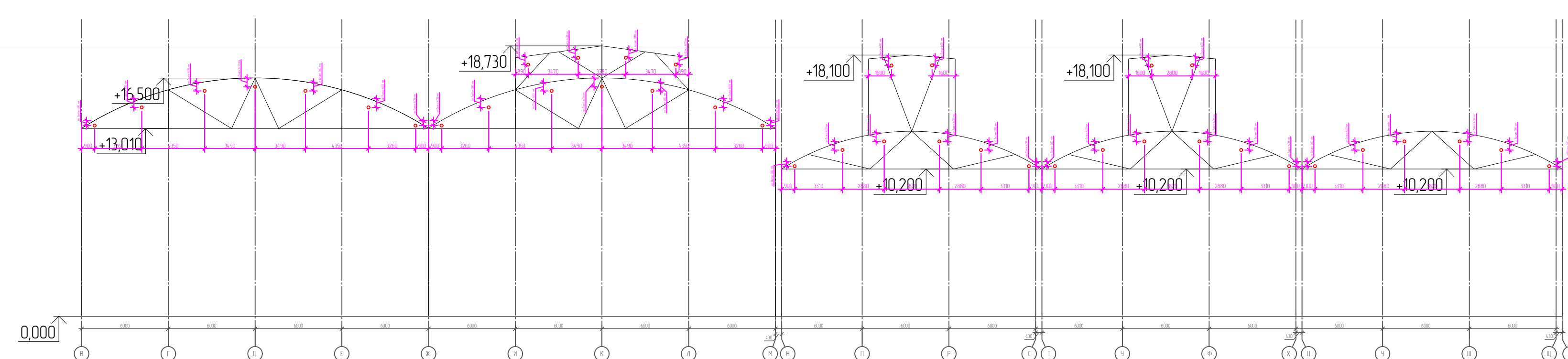
Рарзер 1-1. Расположение лучей С2000-ИПДЛ
