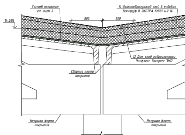
Устройства кровельного покрытия в ендовах
