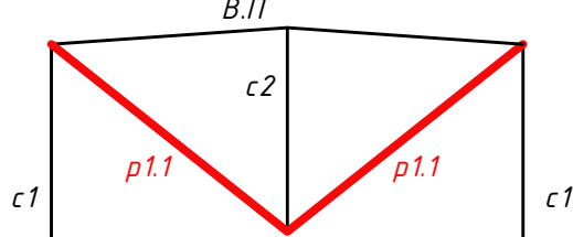
Геометрическая схема ФФ-4.1 с указанием усиливаемых элементов
