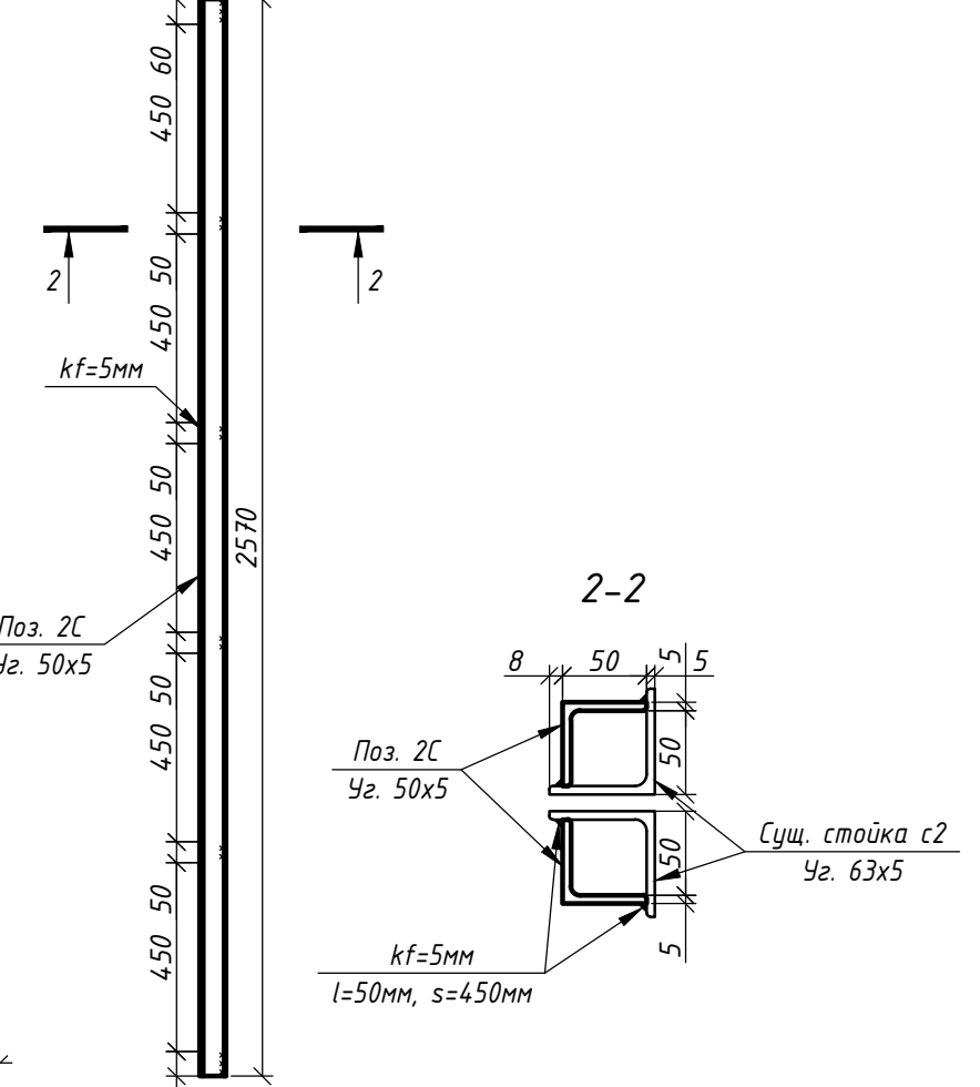
Схема усиления стойки с2
