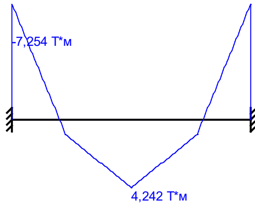
Огибающая величин M_{\max} по значениям расчетных нагрузок
