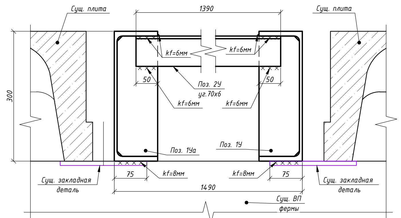
1-1 Стальной каркас
