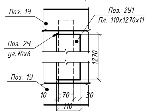
Вид а Стальной каркас
