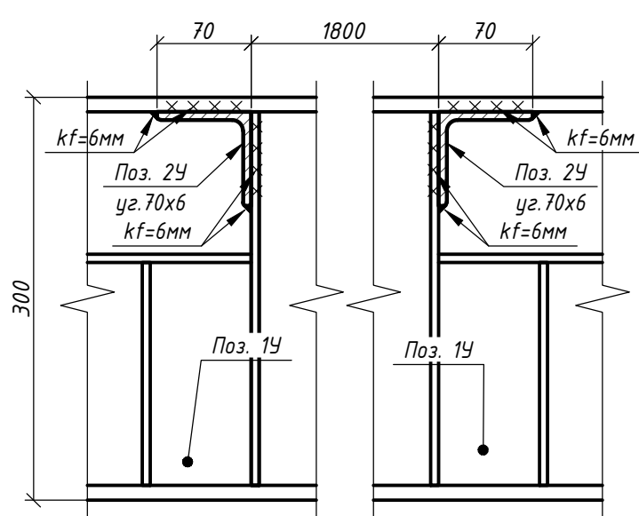
4-4 Стальной каркас
