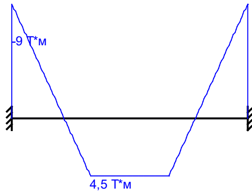
Огибающая величин M_{\max} по значениям расчетных нагрузок
