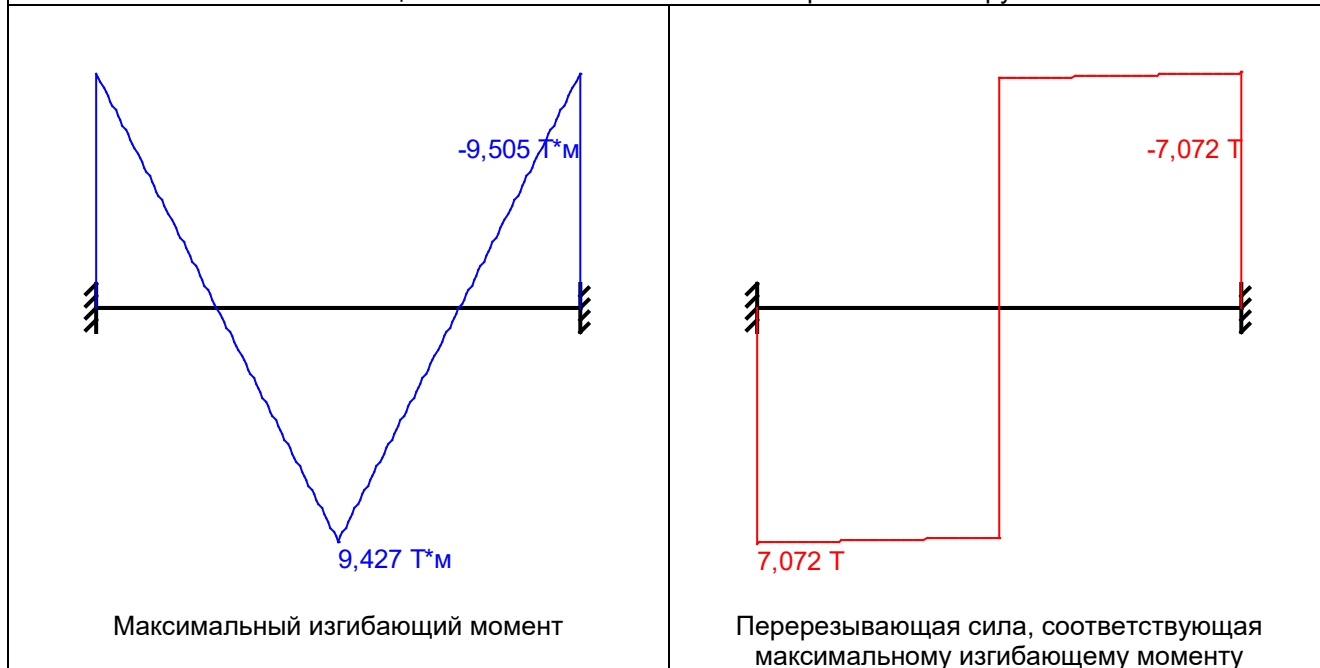
Огибающая величин M_{\max} по значениям расчетных нагрузок
