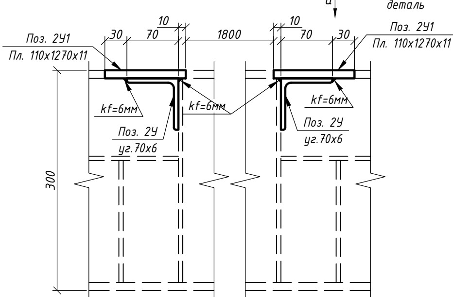
5-5 Стальной каркас
