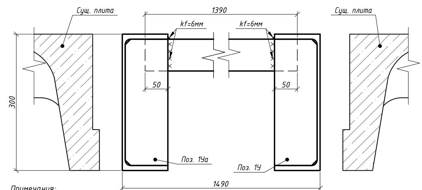
2-2 Стальной каркас
