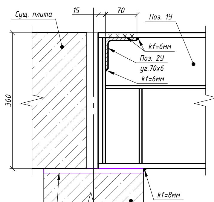
3-3 Стальной каркас
