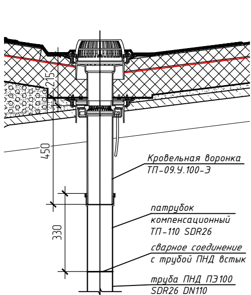
Узел стыковки воронки и трубы
