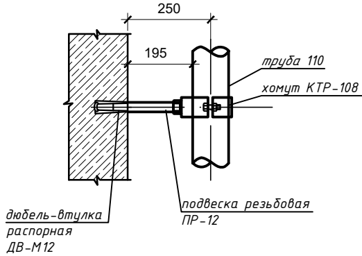
Узел крепления 4
