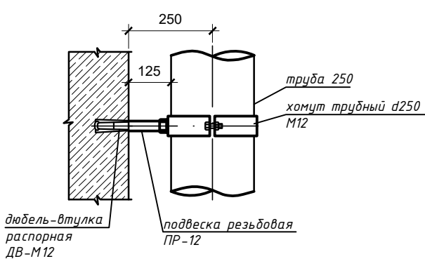
Узел крепления 6
