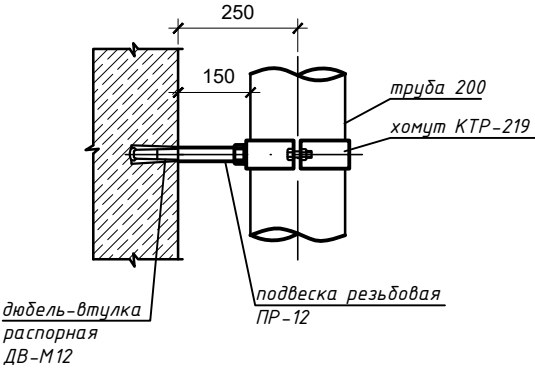
Узел крепления 5
